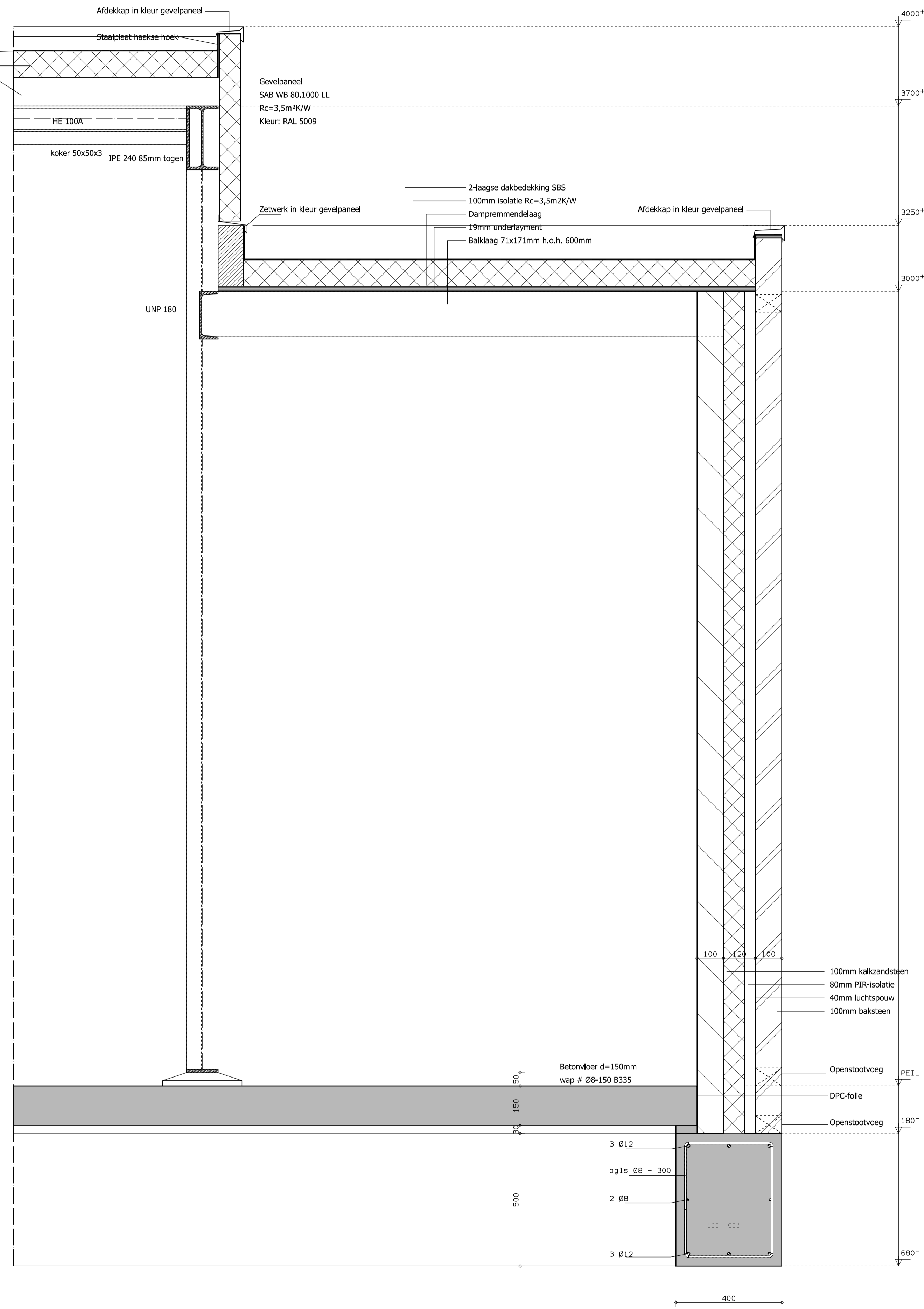
2 - Doorsnede op as-6
